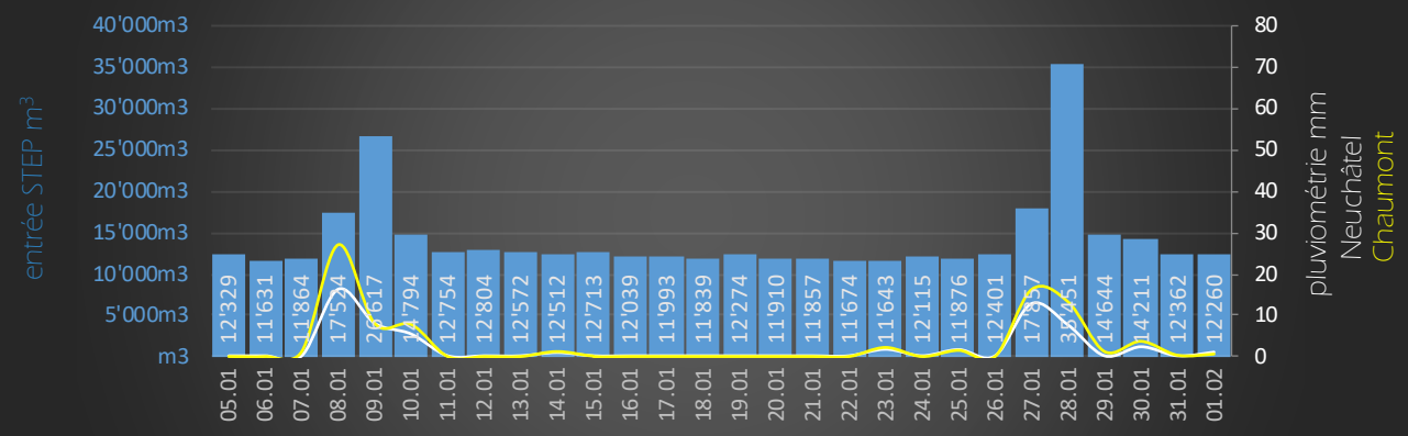
débit d'eau brute sur les 30 derniers jours en m 3 et pluviométrie en mm sur le bassin versant STEP
